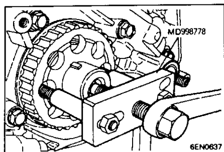
17. 曲轴链轮“B”的拆卸
