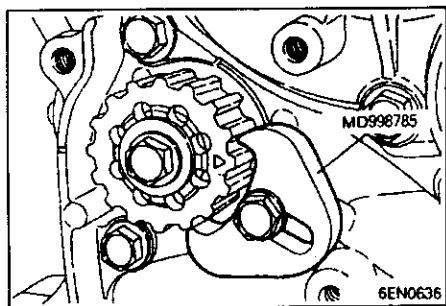
15. 无声轴链轮的拆卸
