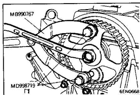
18. 凸轮轴链轮的螺栓的松驰
